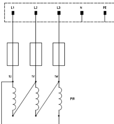
CEE Stecker 5 polig
